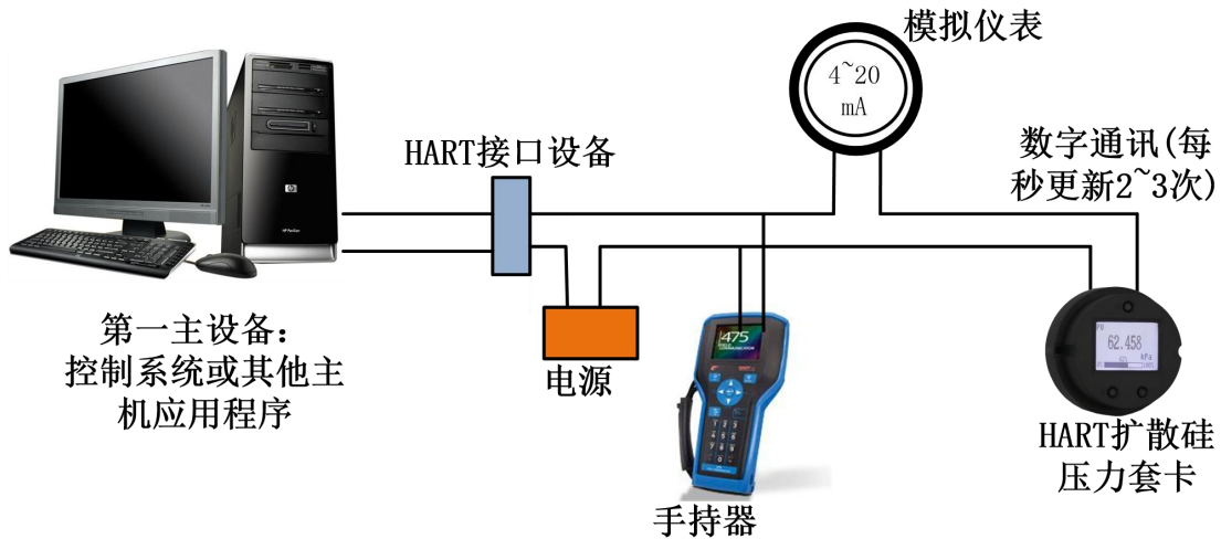
图 4.1 (4~20)mA 兼容模式
