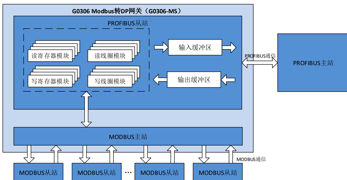
图 6 网关原理框图（G0306-MS）
